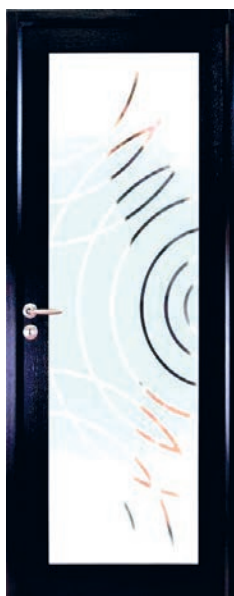
Bloc-porte LM30GV Peint Noir - Vitrage Design V04 2 040 x 830 mm Huisserie H. 72 x L. 58 cm
